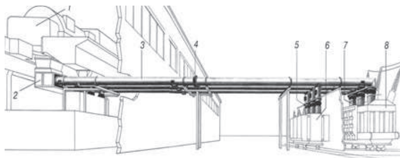
Рис. 1.1 Принципиальное исполнение трассы токопроводов генераторного напряжения на ГРЭС 1 – турбогенератор 2 – узел подсоединения токопровода к генератору, включая блок нуля генератора 3 – главный токопровод 4 – компенсатор линейных расширений 5 – токопровод ответвлений на трансформатор СН 6 – трансформатор СН 7 – узел подсоединения токопровода к силовому трансформатору 8 – трансформатор повышающий
