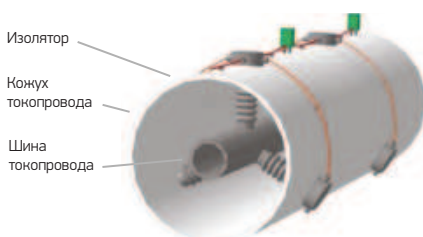
Рис. 1.12 Система контроля изоляции опорных изоляторов – УКОИ
