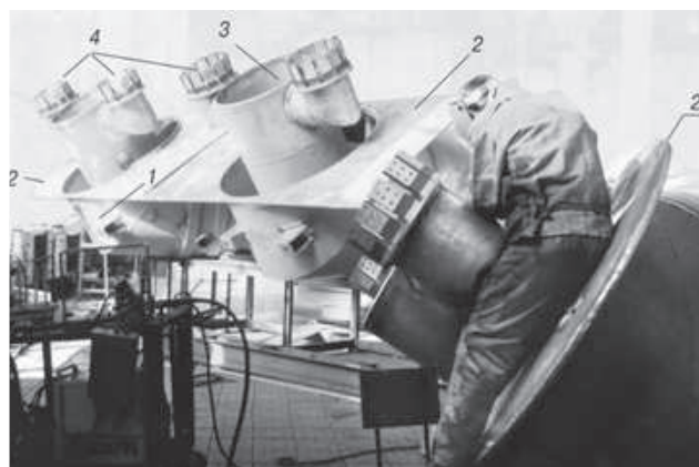
Рис. 1.8 Блок подсоединения токопровода к силовому трансформатору 1 – кожух-экран; 2 – плита переключки экранов; 3 – шина токоведущая; 4 – контактные переходы
