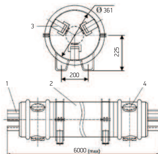
Рис. 3.2 Шинопровод ШЗК-0,4. Секция прямолинейная 1 – шина токоведущая; 2 – оболочка (кожух); 3 – изолятор; 4 – крышка изолятора
