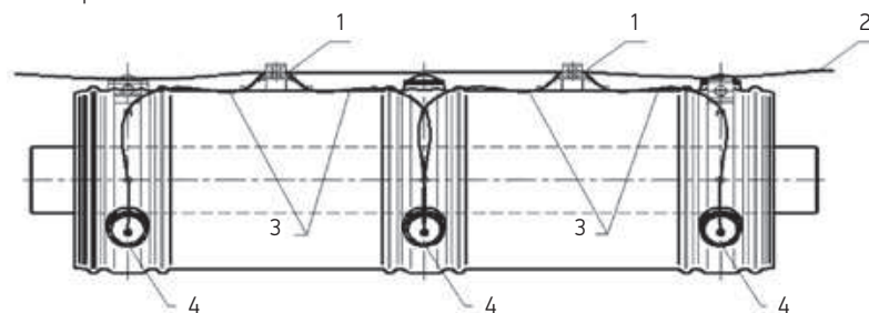
Рис. 1.13 Устройство системы контроля изоляции 1 – блок БМК; 2 – к блоку БОРП; 3 – информационный кабель; 4 – опорный изолятор с датчиком
